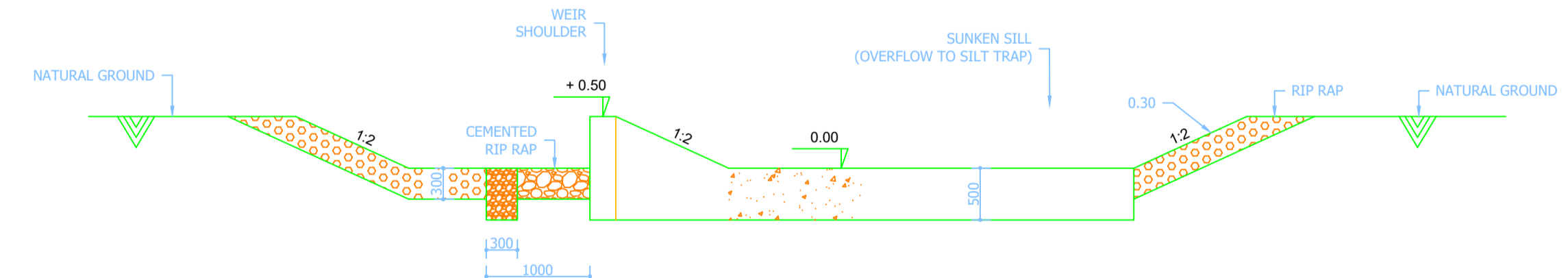
LONGITUDINAL SECTION D-D SCALE 1:50
