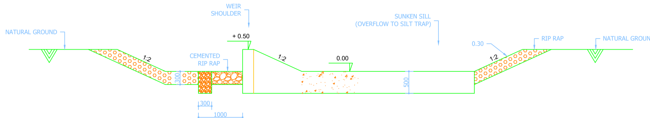
LONGITUDINAL SECTION D-D SCALE 1:50
