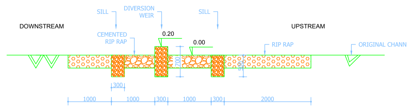
LONGITUDINAL SECTION C-C SCALE 1:50
