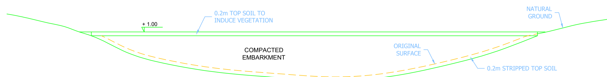
LONGITUDINAL SECTION B-B SCALE: HORZ. 1:400 VERT. 1:100
