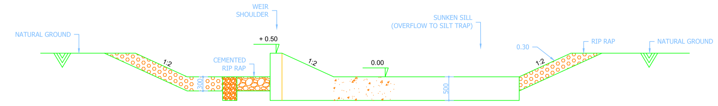
LONGITUDINAL SECTION D-D SCALE 1:50
